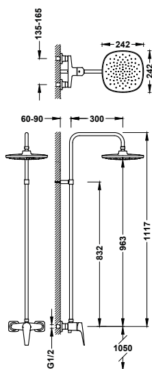
Conjunto de grifo monomando mural de 1 vía para ducha
