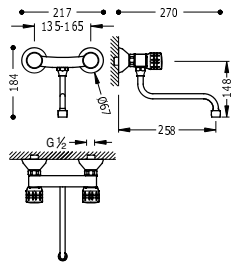
Grifo bimando mural para cocina Con caño inferior. Distancia a pared: 258 mm.
