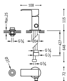
Grifo monomando para bidé con transferencia a duchita Latiguillos de alimentación flexibles G3/8.
