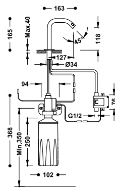
Grifo electrónico de 1 agua con dispensador de jabón automático para lavado
