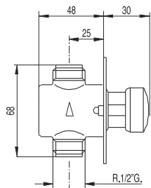
Grifo temporizado empotrado de 1 agua para ducha Entrada y salida con rosca G1/2. Caudal: 16 l/min.
