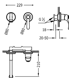
Grifo monomando empotrado para lavabo Cuerpo empotrado incluido e indivisible. Caño de 210 mm.
