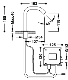
Grifo electrónico de 1 agua para lavado Accionado mediante sensor de infrarrojos.
