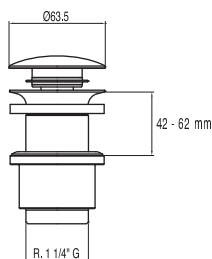
Válvula de desagüe Click-Clack para lavabo sin rebosadero Para encimeras de madera de 42-62 mm. Sin rebosadero. Función Click-Clack. Tapón: Ø 63.5 mm.
