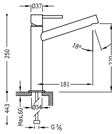
Grifo monomando alto para lavabo Caño largo. Latiguillos de alimentación flexibles G3/8.
