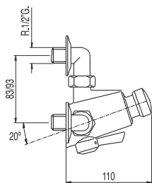
Grifo temporizado mural con selector de temperatura para ducha Entradas opuestas con racores extensibles y válvulas antirretorno. Caudal: 16 l/min.
