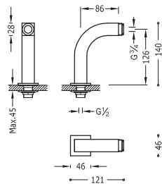
Tomas de agua acodadas de instalación a borde bañera para grifo de bañera
