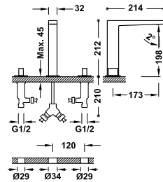
Grifo bimando de repisa para lavabo De instalación libre. Con volantes.
