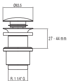
Válvula de desagüe Click-Clack para lavabo sin rebosadero Para encimeras de madera de 27-44 mm. Sin rebosadero. Función Click-Clack. Tapón: Ø 63.5 mm.
