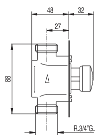
Grifo temporizado empotrado de 1 agua para ducha Entrada y salida con rosca G3/4. Caudal: 20 l/min.
