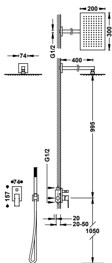
Kit de grifo monomando empotrado de 2 vías para ducha
