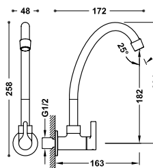
Grifo mural de 1 agua para office o lavadero Con conexión roscada macho de G1/2.
