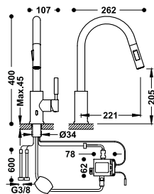
Grifo electrónico con caño extraíble y 2 tipos de chorro para cocina
