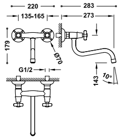
Grifo bimando mural para cocina Con caño inferior. Distancia a pared: 273 mm.
