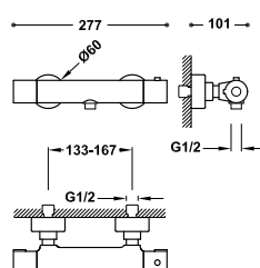
Grifo termostático mural para ducha Ducha de mano anticalcárea: Ø 100 mm. Soporte orientable para ducha de mano. Flexo metálico.
