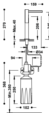
Dispensador electrónico alto de jabón para lavabo y cocina
