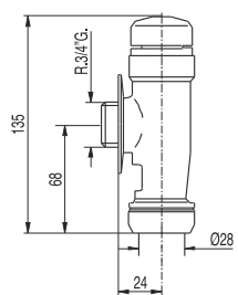
Grifo de descarga temporizado mural de 1 agua para urinario
