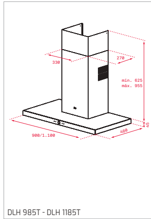
DLH 985T - DLH 1185T
