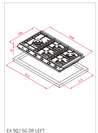
EX 90.1 5G DR LEFT
