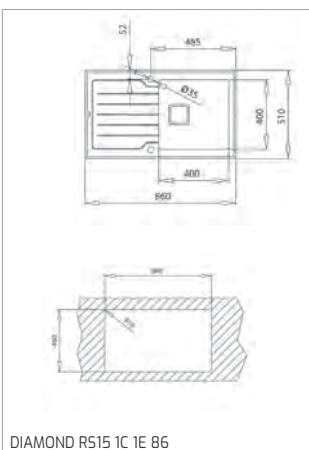
DIAMOND RS15 1C 1E 86
