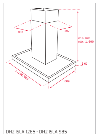
DH2 ISLA 1285 - DH2 ISLA 985
