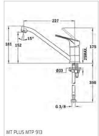
MT PLUS MTP 913
