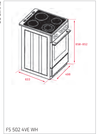
FS 502 4VE WH
