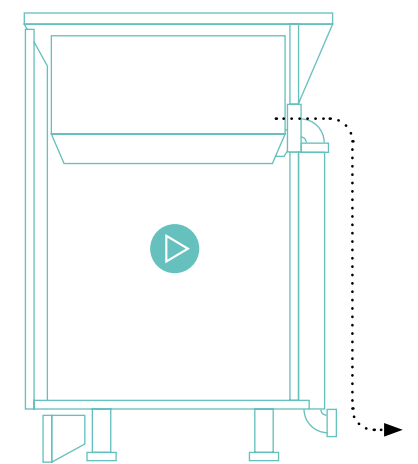
Instalación con salida de aire al exterior
