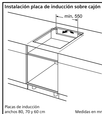
Placas de inducción anchos 80, 70 y 60 cm Medidas en mm
