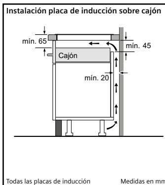
Todas las placas de inducción Medidas en mm
