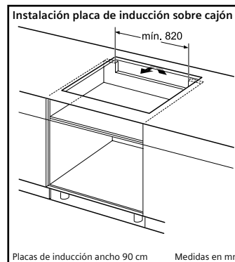
Placas de inducción ancho 90 cm Medidas en mm
