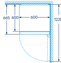
Instalación apertura puerta 90° junto a la pared:
