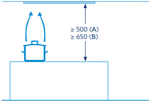
Desde el borde superior de la parrilla: A: placa eléctrica mín. 500 mm B: placa de gas mín. 650 mm
