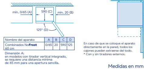
Instalación apertura puerta 125° enrasado con los muebles:
