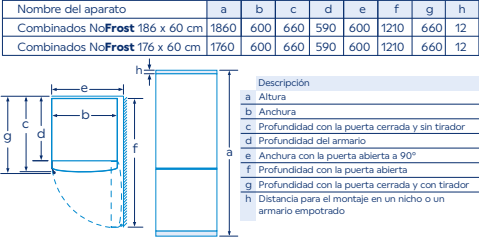
Modelos: 3KFE551MI, 3KFE551WI, 3KFE351MI y 3KFE351WI Instalación apertura puerta 90° junto a la pared:
